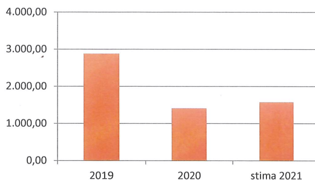
Figura 11. Consumi di metano Tratos SRL nel triennio 2019-2021
