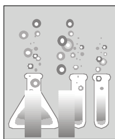
EN 50267 IEC 60754
