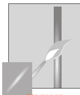
EN 50265 IEC 60332-1
