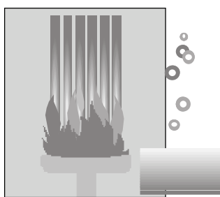
EN 50266 IEC 60332-3
